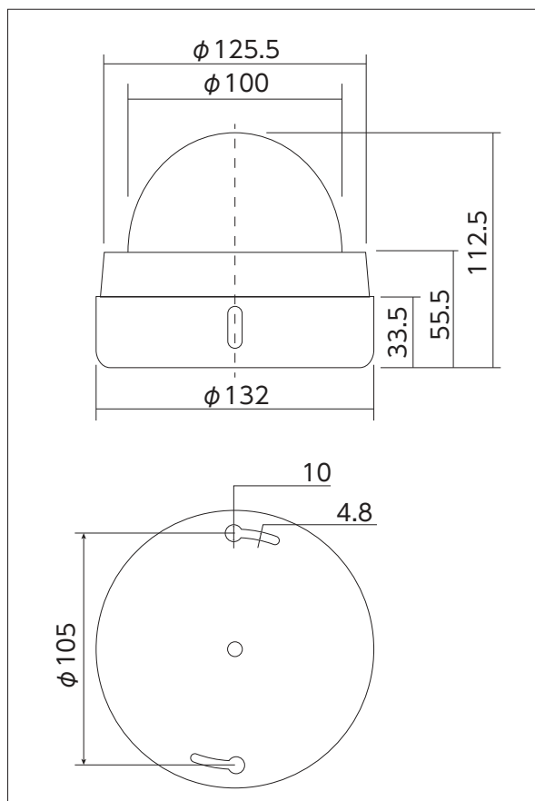
製品寸法図(単位:mm)
